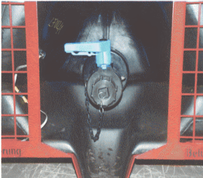
Abb. 4: Leitfähiges Bodenventil mit Erdungskabeln
