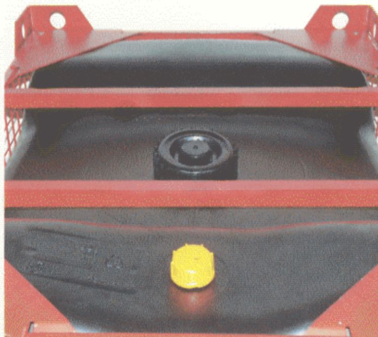
Abb. 2: Ansicht der Containeroberseite
