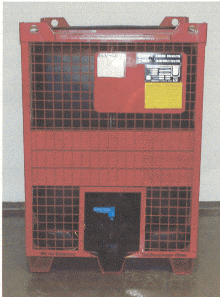
Abb. 3: Gesamtansicht des Prüfmusters
