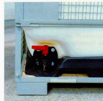
Vollständige Restentleerbarkeit durch schrägen Unterboden
